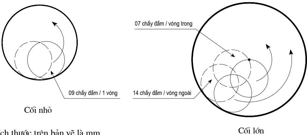
Hình 3. Sơ đồ bố trí chày đầm
