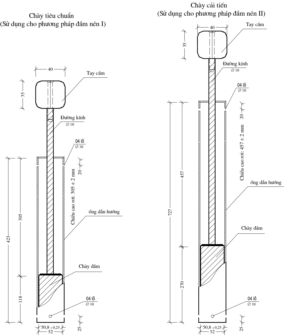
Hình 3. Sơ đồ bố trí chày đầm
